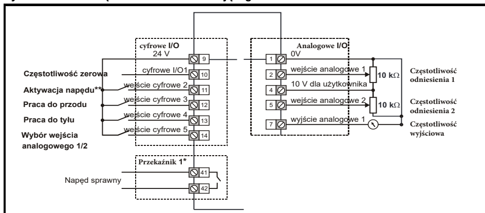
Rysunek 6-3 Połączenia terminala sterującego Commander C200 / C300
