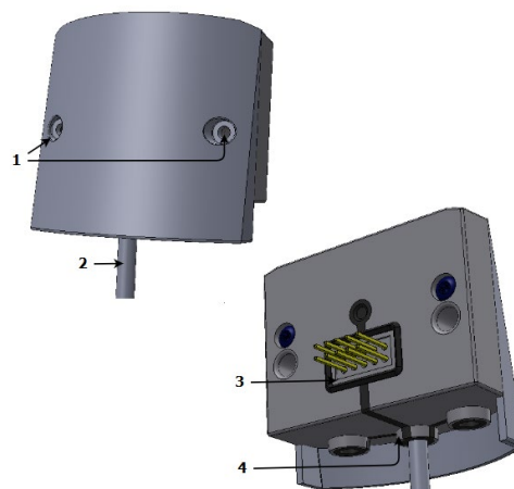
Rysunek 6. Budowa modułu APT-ELF2-USB-1
