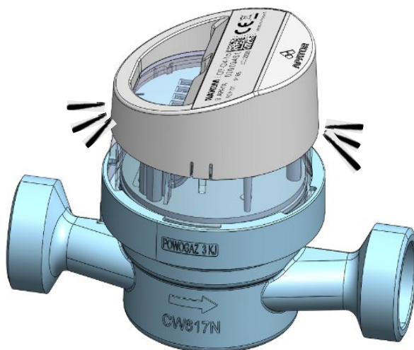
Rys. 3. Widok na zmontowany wodomierz JS Smart + z nakładką OP-04-1a.
