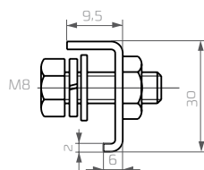
zacisk 16 - 120 mm 2
