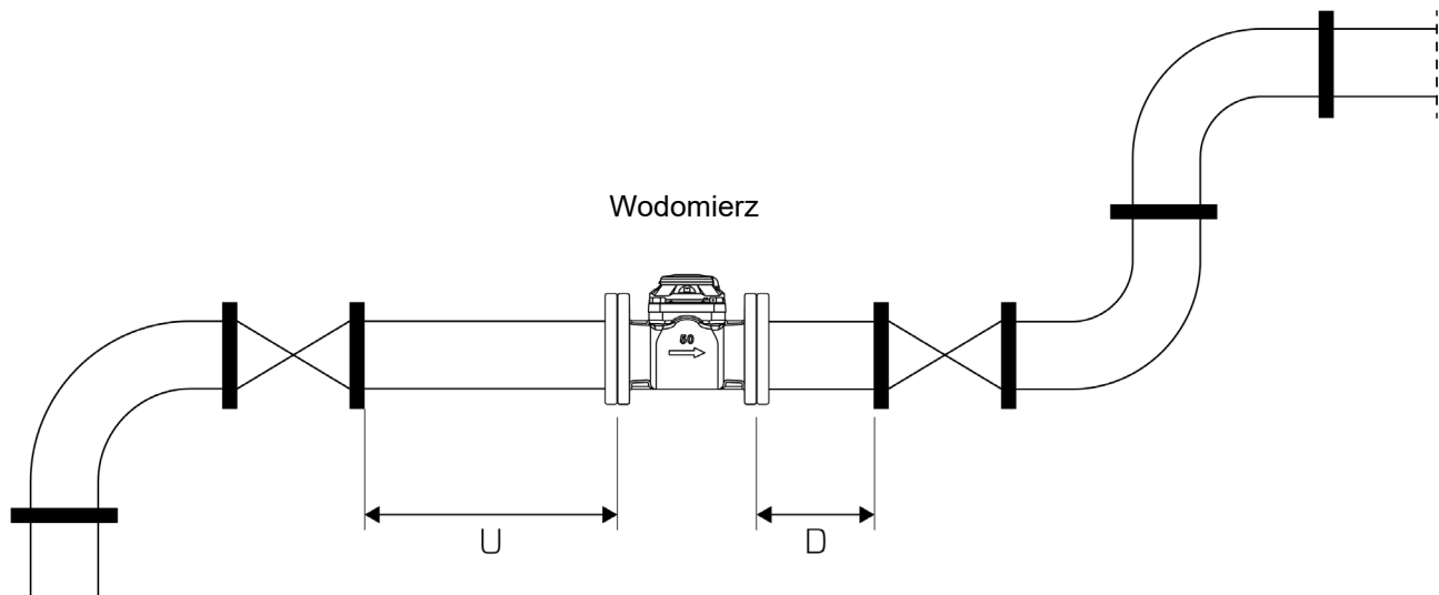
Rys. 2. Zabudowa wodomierza.
