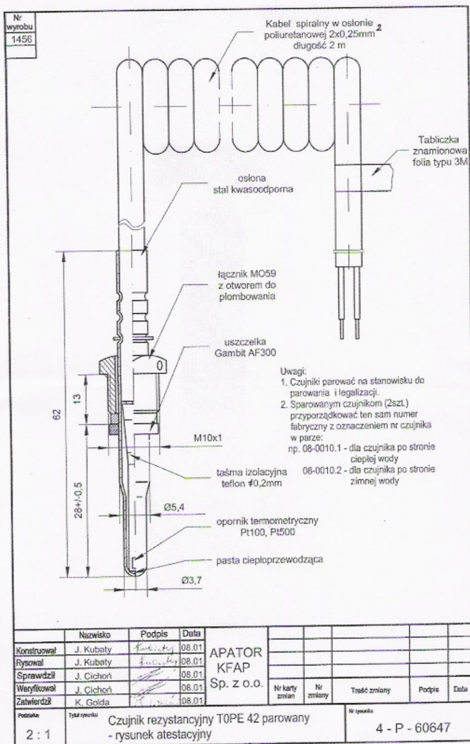
Rysunek 1. Czujnik rezystancyjny TOPE 42 parowany - rysunek atestacyjny.
